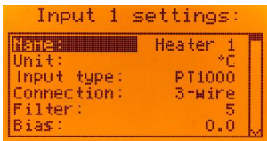
„Input settings” menu
